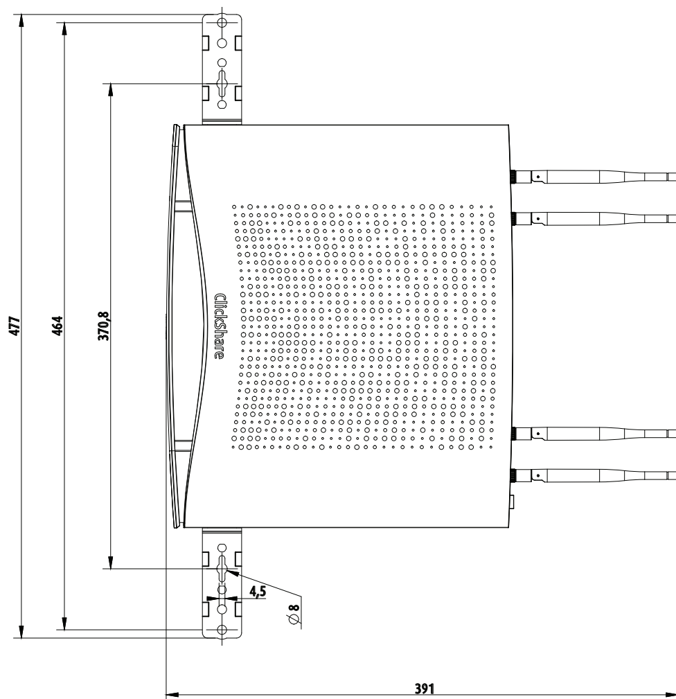
画像 4-2 取り付け穴の寸法
