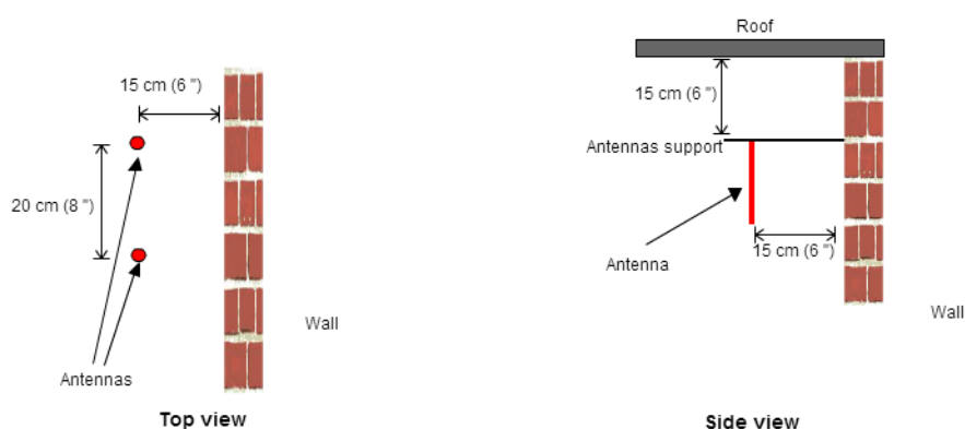
画像 4-5 会議室に取り付けたアンテナの詳細図
