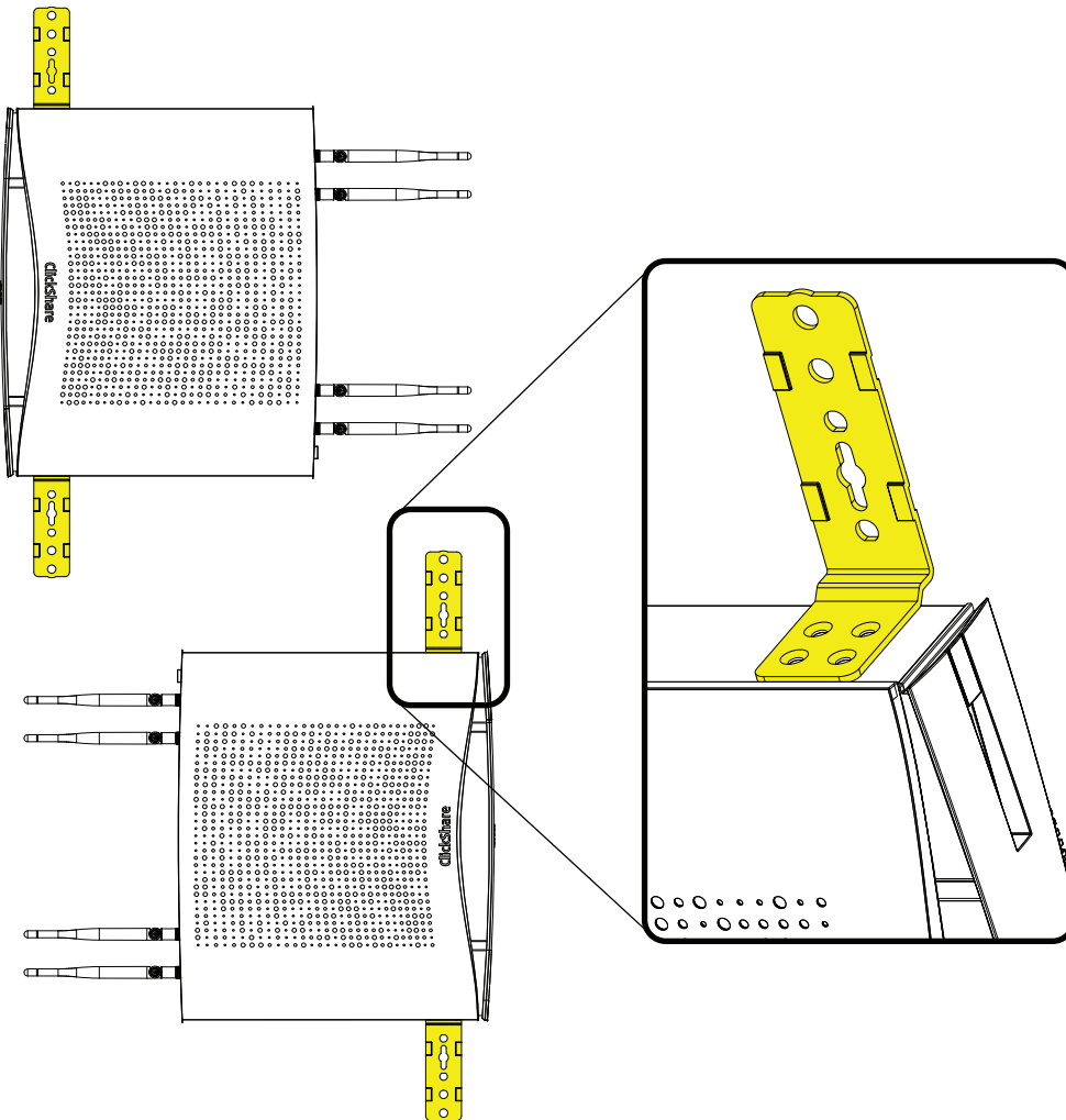
画像 4-1 取り付け金具
