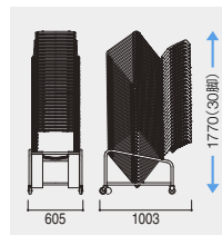
チェアポーターP型に30脚スタッキングできます。
